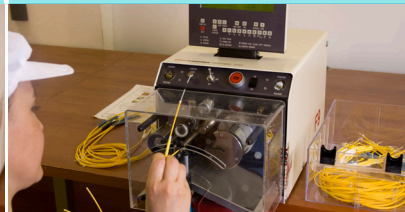
Kabel Abmantelung
