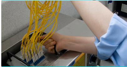
Steckverbinder Oberflächenreinigung
