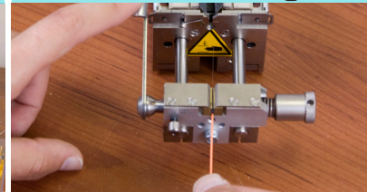
Faser Abmantelung
