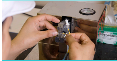
Serrage de Connecteur
