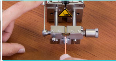
Décapage de la fibre
